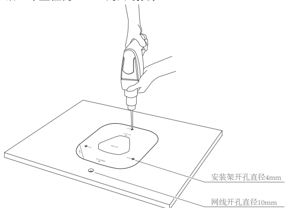
图3-3 钻孔示意图
