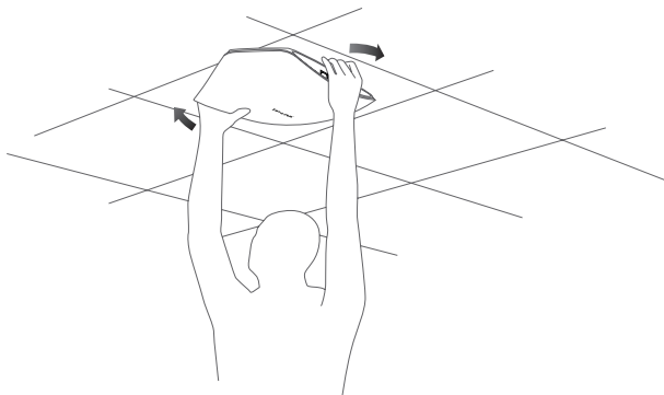
图3-7 吸顶安装完成示意图
